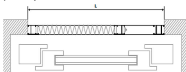
Montaż bezpośrednio do muru
