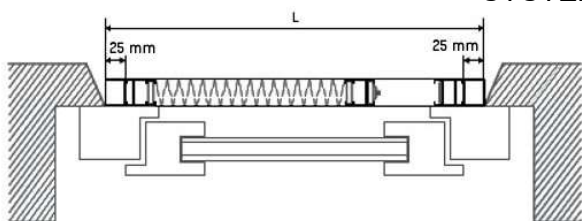
Montaż bezpośrednio do ościeżnicy (zalecany jest profil dodatkowy, który należy uwzględnić przy zamawianiu)
